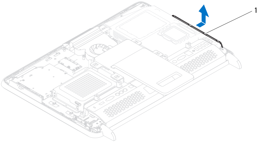
1 boèni U/I poklopac
