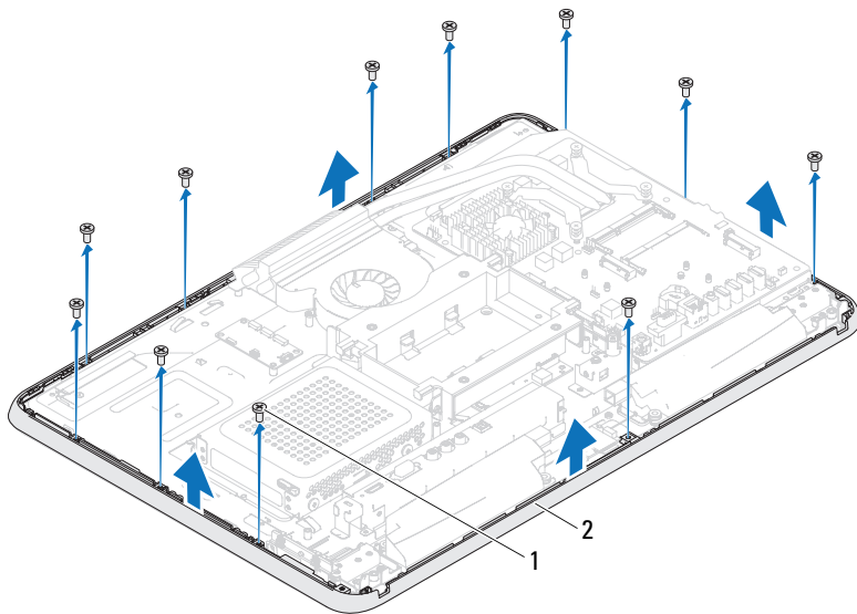
1 zavrtnji (11) 2 srednji okvir
